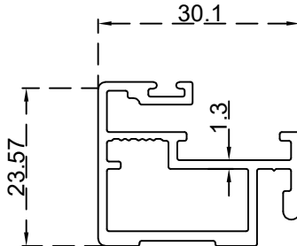
برواز كيبس 36 ملم الرقم التسلسلي للصنف: BLT4457 الوزن 0.254:(Kg/m)
