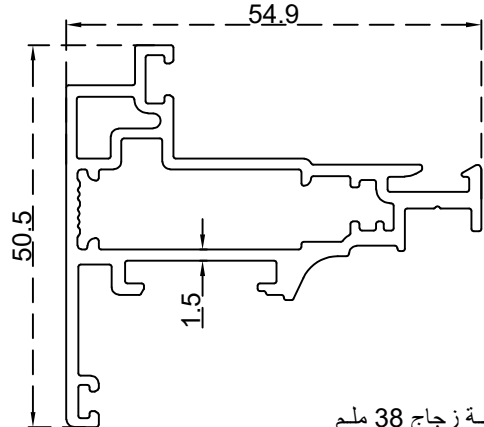
دفة زجاج 38 ملم الرقم التسلسلي للصنف: BLT4484 الوزن 0.981:(Kg/m)
