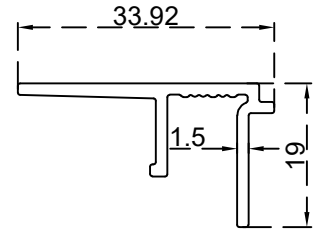
حامل زجاج ثابت الرقم التسلسلي للصنف: BLT4478 الوزن 0.277:(Kg/m)
