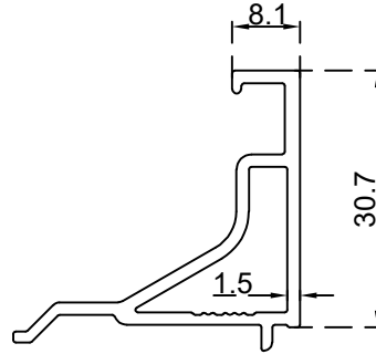
كليبس ثابت زجاج 42 ملم الرقم التسلسلي للصنف: BLT4464 الوزن 0.431:(Kg/m)
