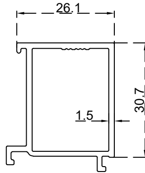
كليبس ثابت زجاج 24 ملم الرقم التسلسلي للصنف: BLT4472 الوزن 0.477:(Kg/m)
