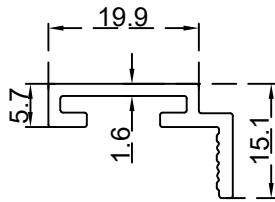
برواز 20 ملم الرقم التسلسلي للصنف: BLT4479 الوزن 0.230:(Kg/m)
