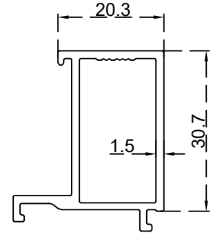
كليبس ثابت زجاج 30 ملم الرقم التسلسلي للصنف: BLT4471 الوزن 0.468:(Kg/m)
