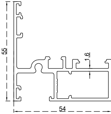
قاطع زجاج 16 ملم الرقم التسلسلي للصنف: BLT4454 الوزن 1.043:(Kg/m)
