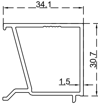
كليبس ثابت زجاج 16 ملم الرقم التسلسلي للصنف: BLT4462 الوزن 0.507:(Kg/m)
