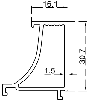
كليبس ثابت زجاج 34 ملم الرقم التسلسلي للصنف: BLT4473 الوزن 0.451:(Kg/m)
