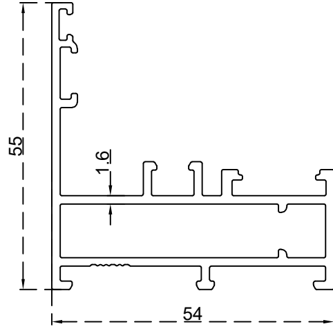
حلق 25 ملم الرقم التسلسلي للصنف: BLT4452 الوزن 0.986:(Kg/m)
