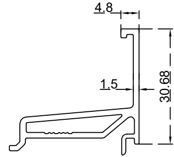
كليبس ثابت زجاج 45 ملم الرقم التسلسلي للصنف: BLT4463 الوزن 0.437:(Kg/m)
