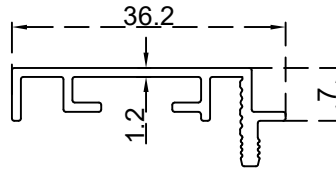
برواز كيبس 36 ملم الرقم التسلسلي للصنف: BLT4457 الوزن 0.254:(Kg/m)
