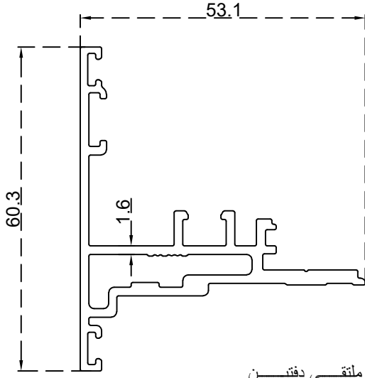
ملتقى دفتين الرقم التسلسلي للصنف: BLT4474 الوزن 0.927:(Kg/m)
