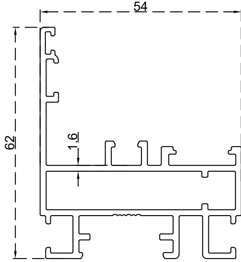
حلق منوبلوك 30 ملم الرقم التسلسلي للصنف: BLT4451 الوزن 1.180:(Kg/m)
