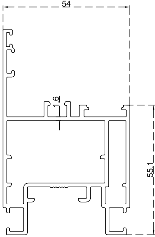
حلق منوبلوك 55 ملم الرقم التسلسلي للصنف: BLT4466 الوزن 1.579:(Kg/m)
