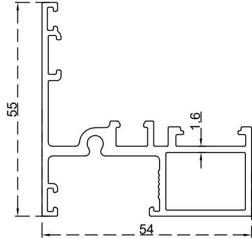
قاطع زجاج 24 ملم الرقم التسلسلي للصنف: BLT4455 الوزن 1.022:(Kg/m)
