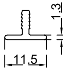
تي تسكيرة الرقم التسلسلي للصنف: BLT3660 الوزن 0.086:(Kg/m)
