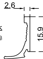
كابيس دفة الرقم التسلسلي للصنف: BLT4465 الوزن 0.123:(Kg/m)
