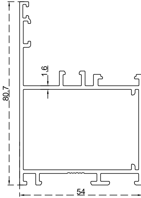
حلق 50 ملم الرقم التسلسلي للصنف: BLT4453 الوزن 1.263:(Kg/m)
